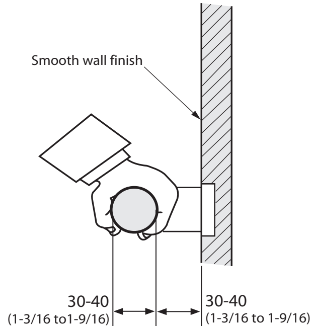
Figure 4.2.10.1 Grab Bar
