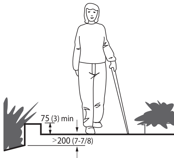
Figure 4.1.4.1 Edge Protection
